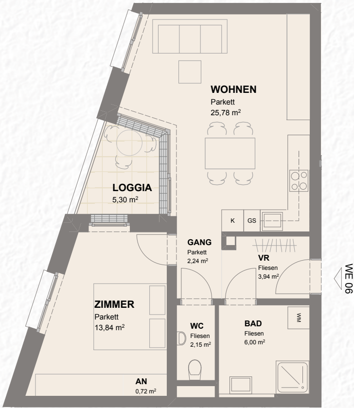
GRUNDRISS TOP 06 – 1:100
