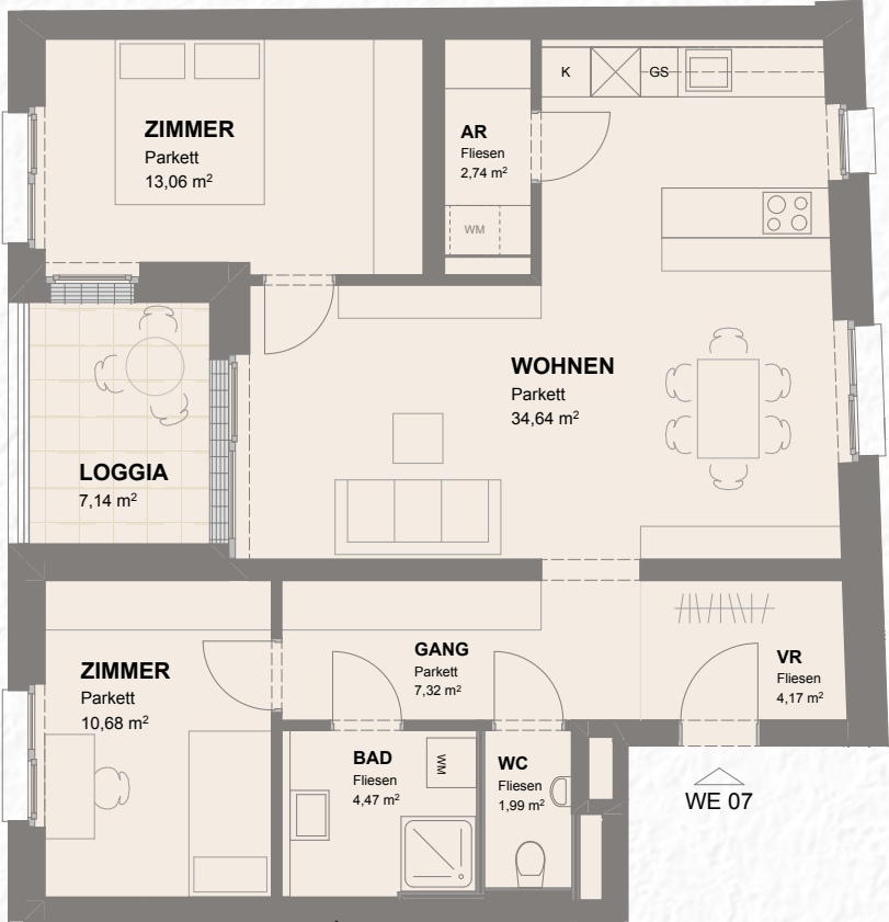
GRUNDRISS TOP 07 – 1:100
