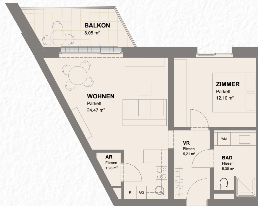
GRUNDRISS TOP 06 – 1:100
